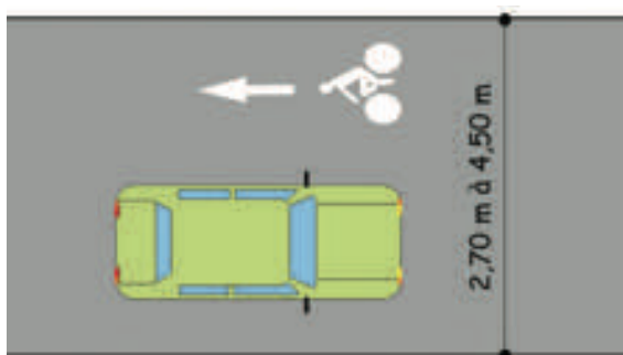
Marquage non séparatif d'un double-sens cyclable
